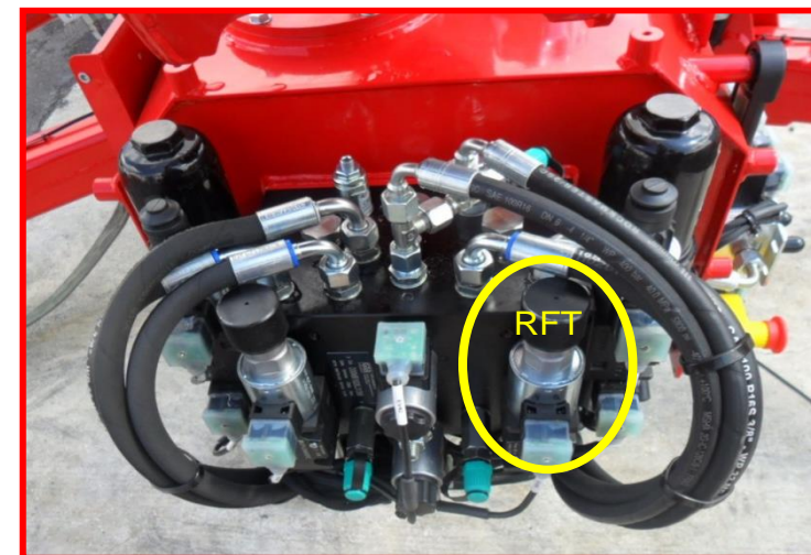
Afbeelding 26: klep rechts van de filtergroep.
