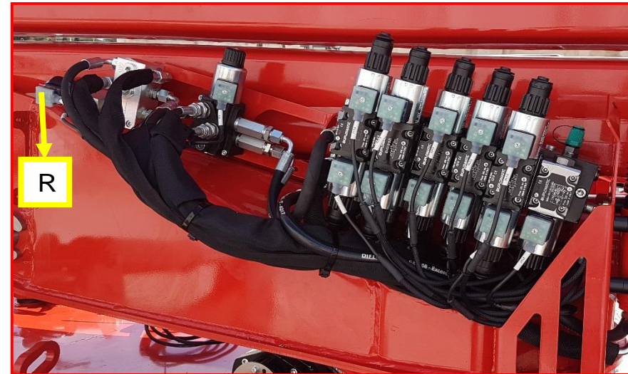
Afbeelding 23a: noodbedieningseenheid op de toren als met een momentbegrenzer (*optioneel).
