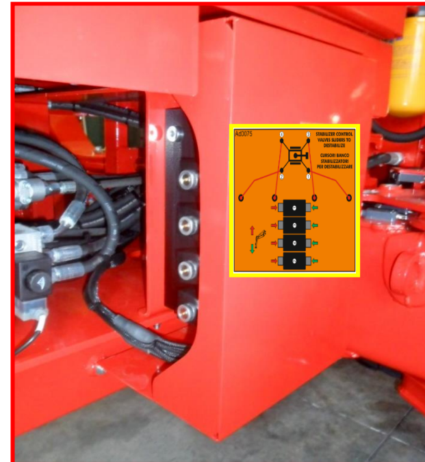
Afbeelding 36: bedieningspaneel stempelpoten.
